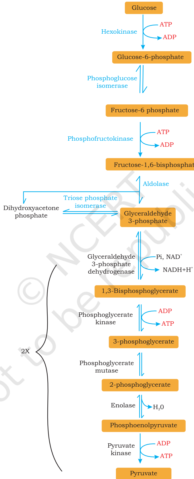
Fig. 5.4: Glycolysis
