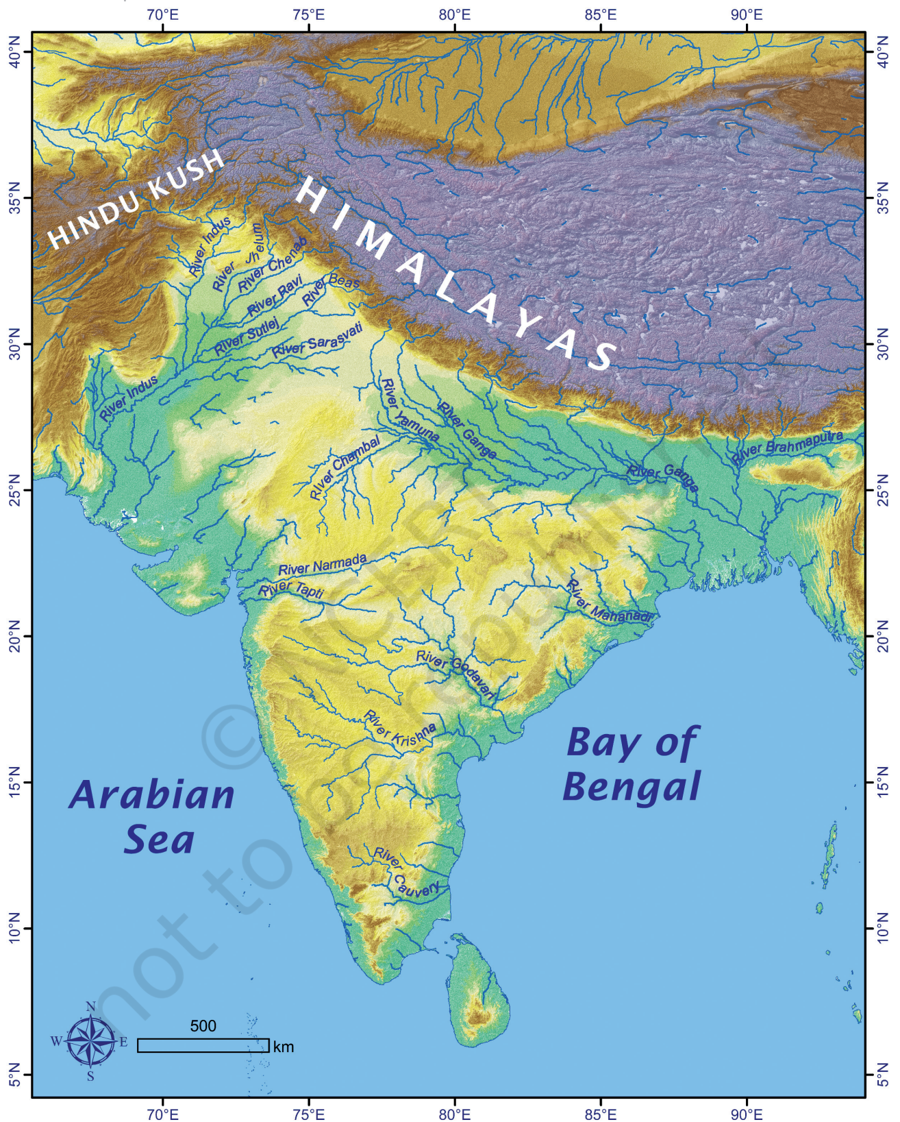
ଚିତ୍ର ୫.୨ । ଭାରତୀୟ ଉପମହାଦେଶର ଏକ ଭୌତିକ ମାନଚିତ୍ର, ଏହାର କିଛି ନଦୀ ସହିତ ।
